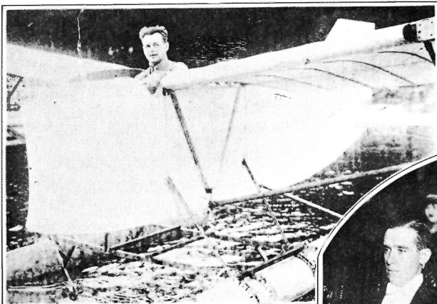
ALEMANIA. —Hidroplano sin motor construido por el famoso aviador Hens Richter, que lo tripula. Richter ha probado su aparato sobre el lago Havel y se propone volar en él desde Francia a Inglaterra, sobre el Canal de la Mancha.
